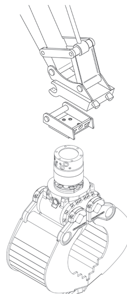
Chwytek z wkręcany adapterem do zamocowania do systemu szybkiej wymiany
