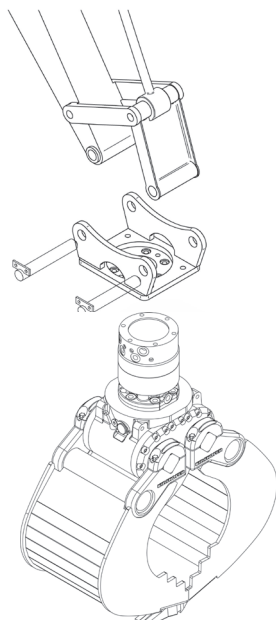
Chwytek z uchwytem do montażu na stałe
