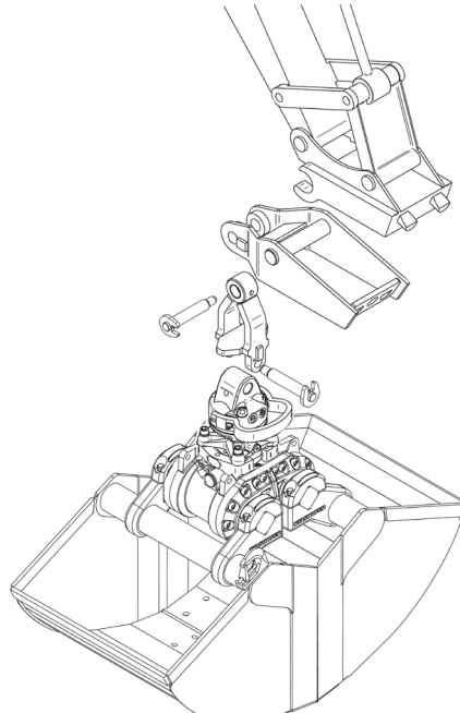
Chwytnak z zawieszeniem przegubowym i systemem szybkiej wymiany
