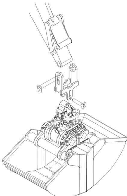
Chwytnak z zawieszeniem przegubowym
